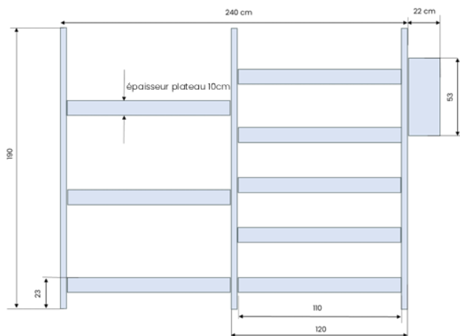
Vue de face Étagère Skalex double
