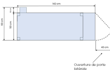
Vue de dessus Étagère Skalex
