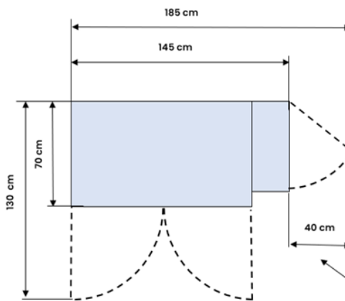
Vue de dessus Armoire Skalex
