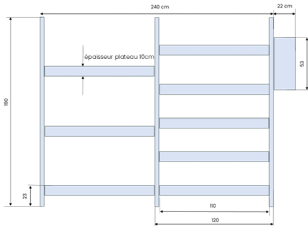
Vue de face Étagère Skalex double
