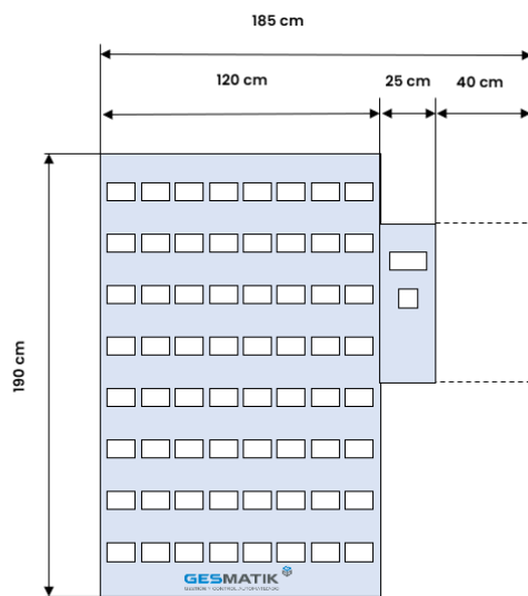
Vue de face Armoire Skalex
