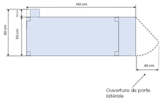
Vue de dessus étagère Skalex
